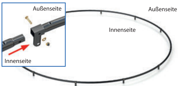
Abb. 1: Zusammenbau des Trampolinrahmens
