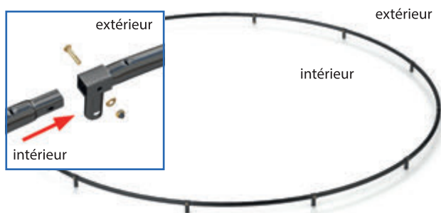
fig. 1 : Assemblage du cadre du trampoline
