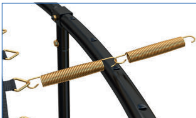
Abb. 4: Einspannen der Feder mit Hilfe einer anderen Feder
