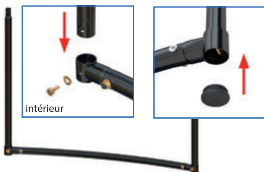
fig. 3 : Assemblage des pieds
