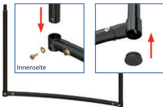
Abb. 3: Zusammenbau der Standfüße
