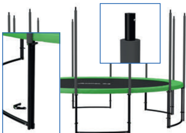
fig. 4: Fixation des montants du filet à l'aide de bagues
