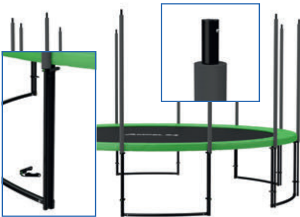
Abb. 4: Befestigung der Netzpfoستen mit den Manschetten
