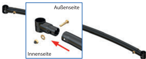
Abb. 2: Zusammenbau der Standfüße
